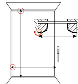
Zalecany pomiar żaluzji z mocowaniami standardowymi
